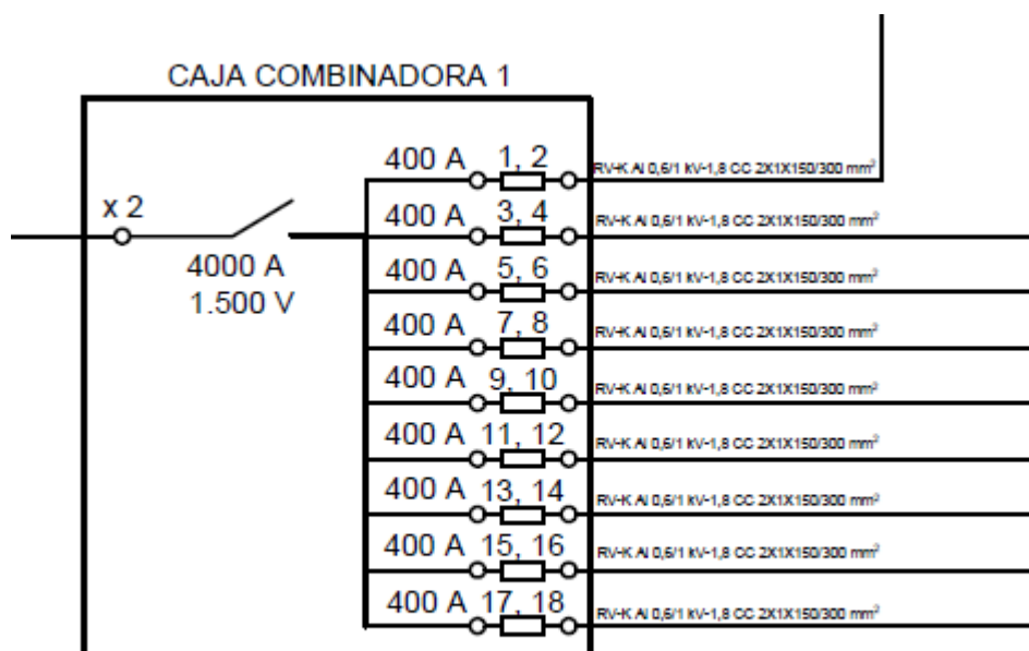
Figura 22.- Cuadro agrupación CC inversor
